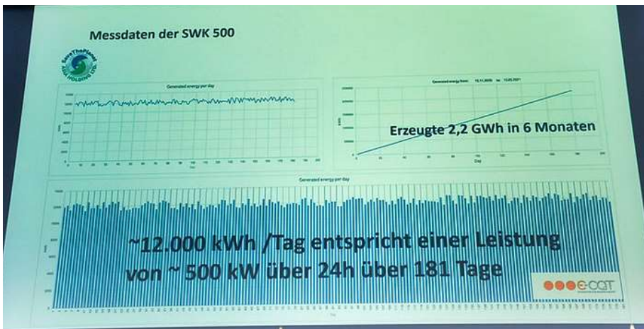
Reale Messdaten des in Thailand laufenden 500-kW-Auftriebskraftwerks.
