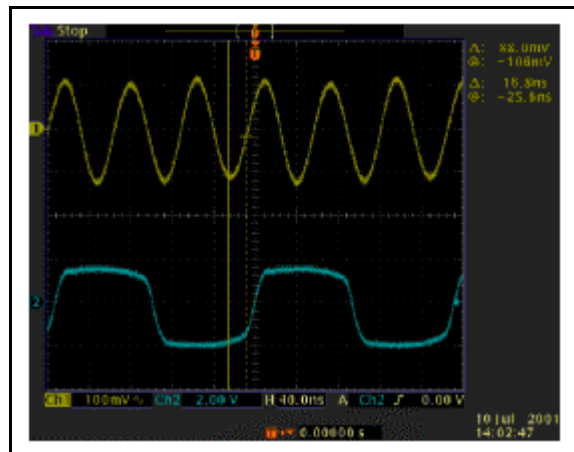
Abbildung 11: LED nur auf Senderplatine
