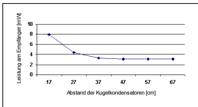
Abbildung 4: Entfernungsabhängigkeit der am Empfänger gemessenen Leistung
