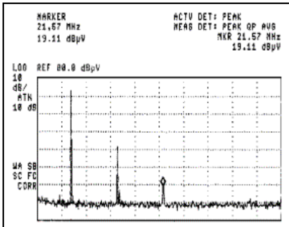
Abbildung 10: Schaltung ohne LED's
