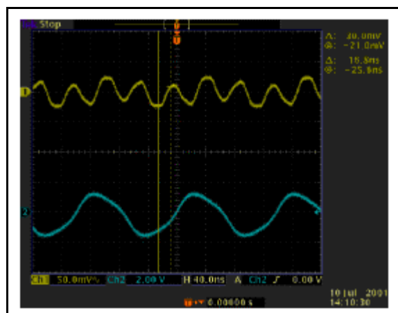
Abbildung 12: LED nur auf Empfängerplatine
