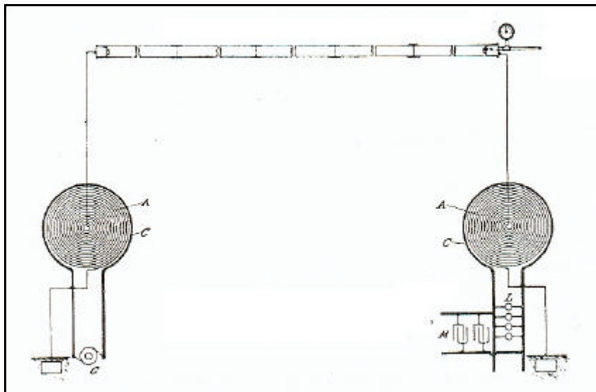
Abbildung 1: Anordnung für Energieübertragung durch eine mit Luft gefüllte Glasröhre, wobei der Luftdruck stark reduziert ist. (Quelle: N. Tesla Colorado Spring Notes 1899-1900)
